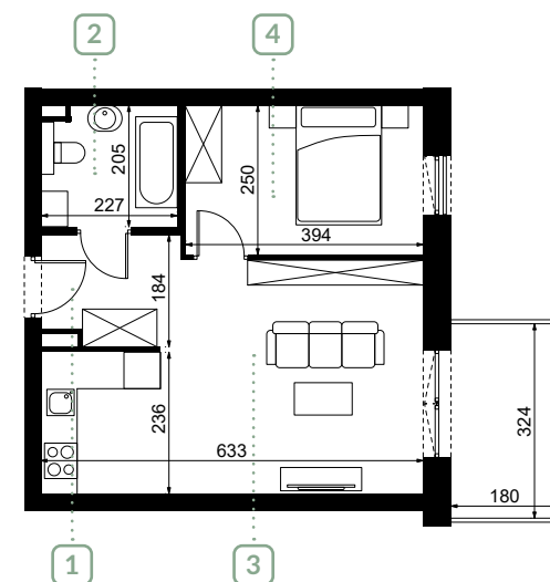
Rzut mieszkania 1.01
