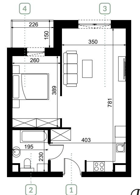
Rzut mieszkania 1.13
