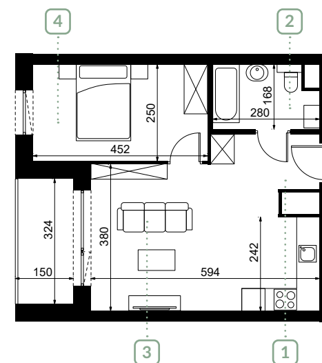
Rzut mieszkania 1.17
