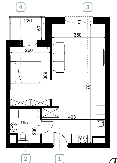
Rzut mieszkania 1.20
