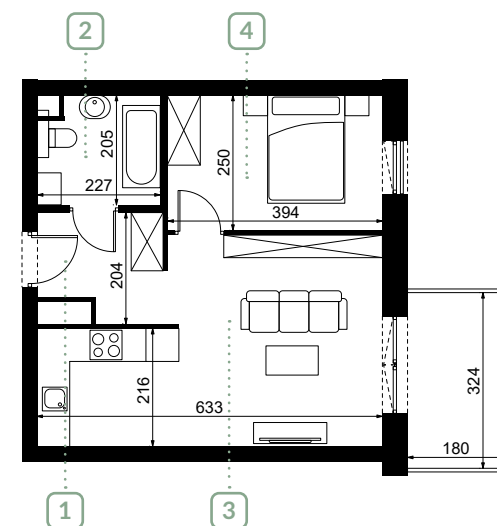
Rzut mieszkania 1.22
