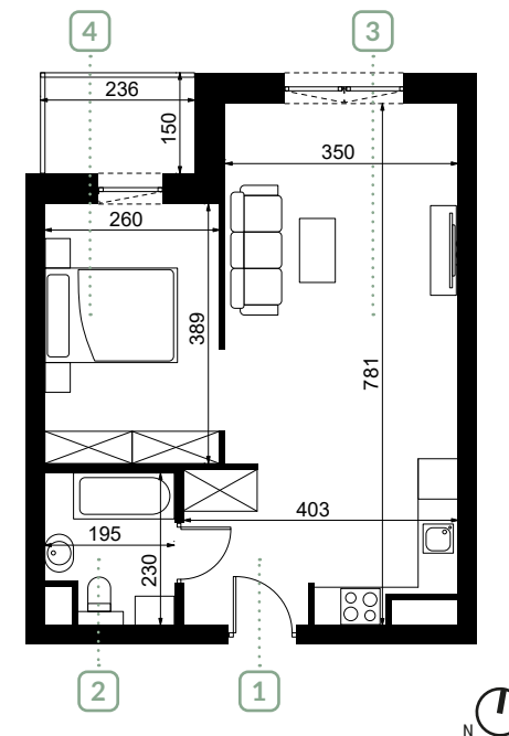
Rzut mieszkania 1.25
