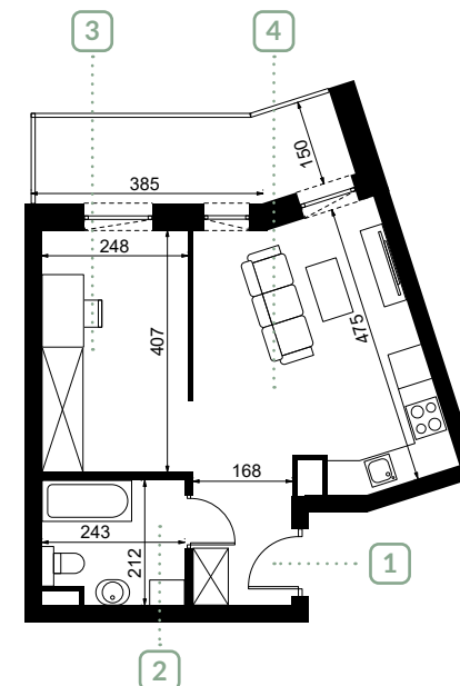
Rzut mieszkania 2.06
