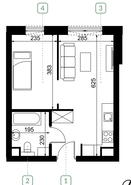
Rzut mieszkania 2.07
