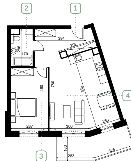
Rzut mieszkania 2.17
