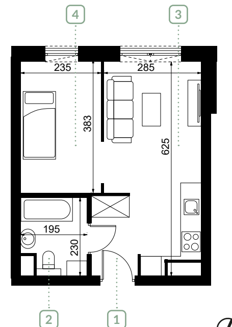
Rzut mieszkania 2.19
